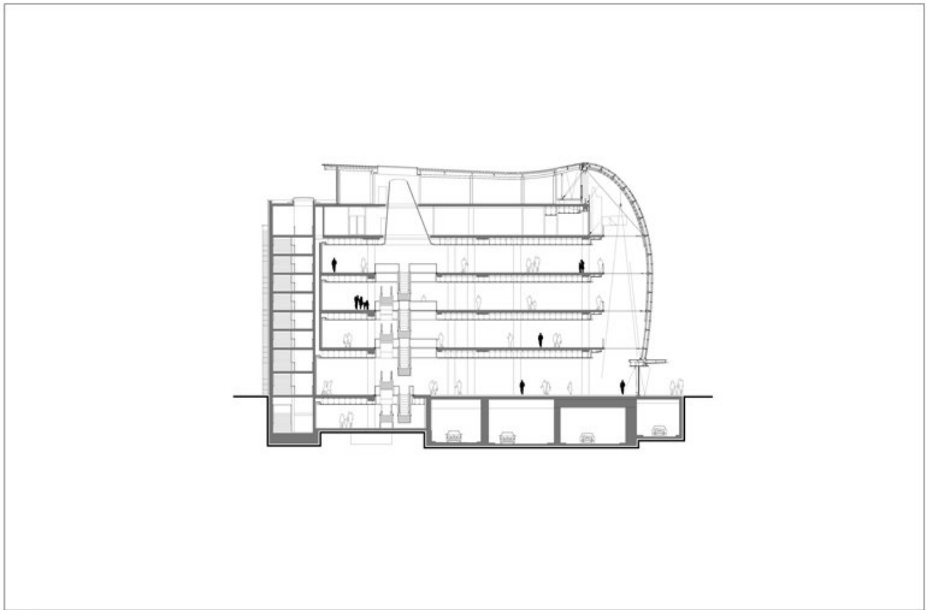
GEBÄUDESCHNITT KAUFHAUS, P & C, KÖLN
