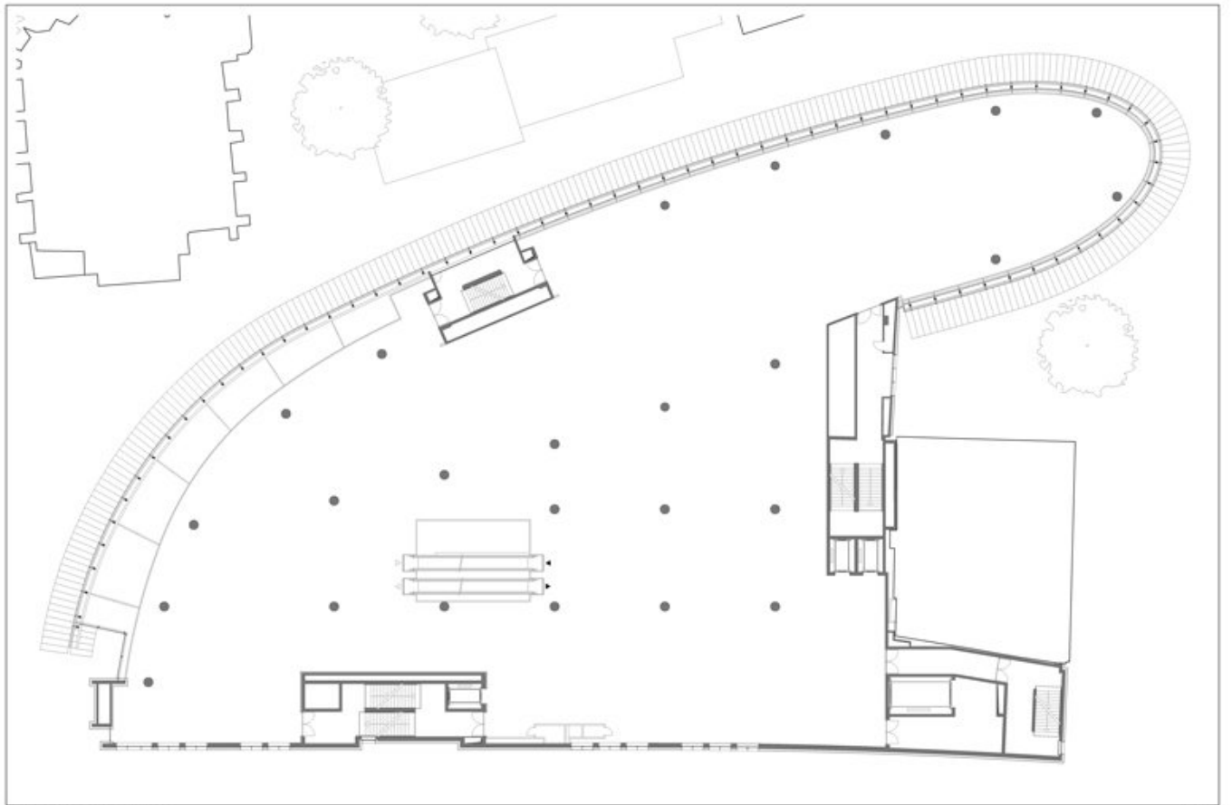
VERKAUFGESCHOSS KAUFHAUS, P & C, KÖLN
