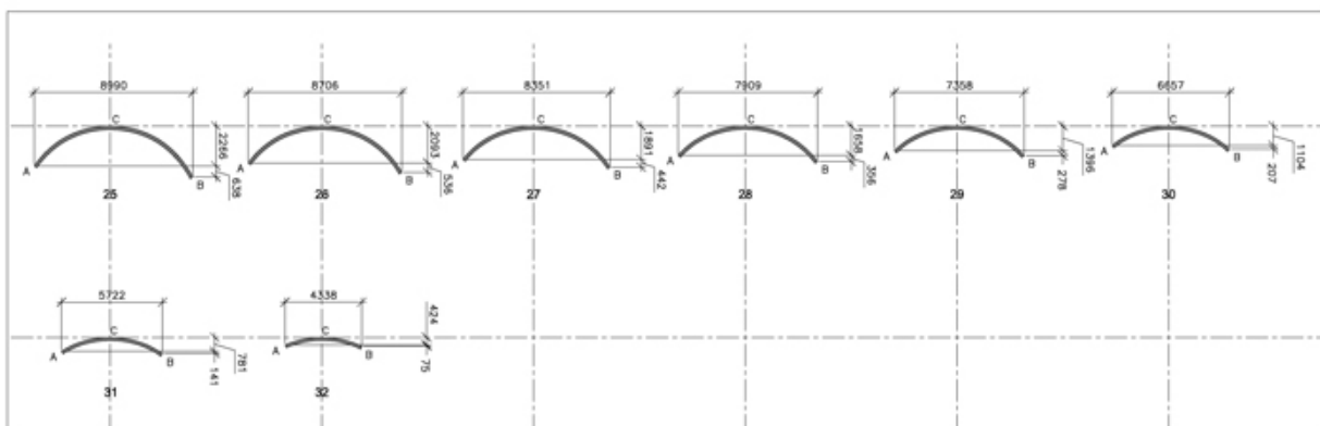
EPU 03A - PLAN D'ÉPURE - Ech : 1/200
