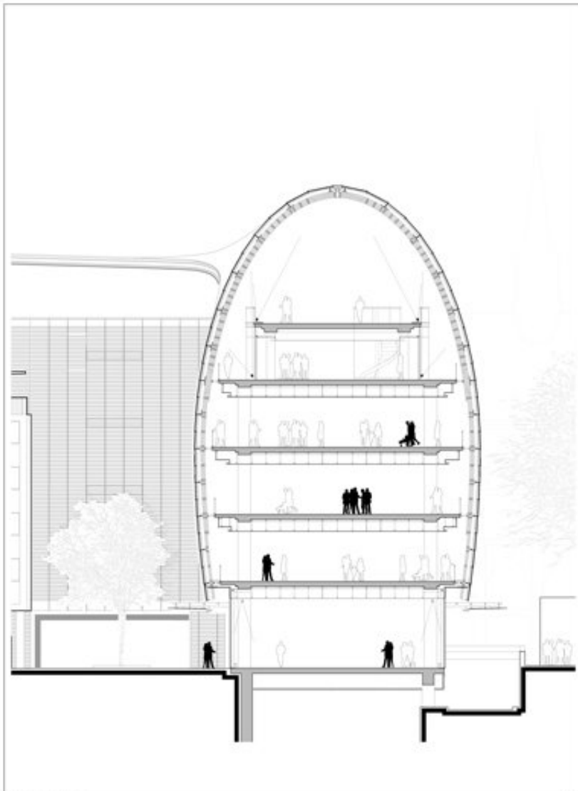
SCHNITT KUPPEL KAUFHAUS, P & C, KÖLN
