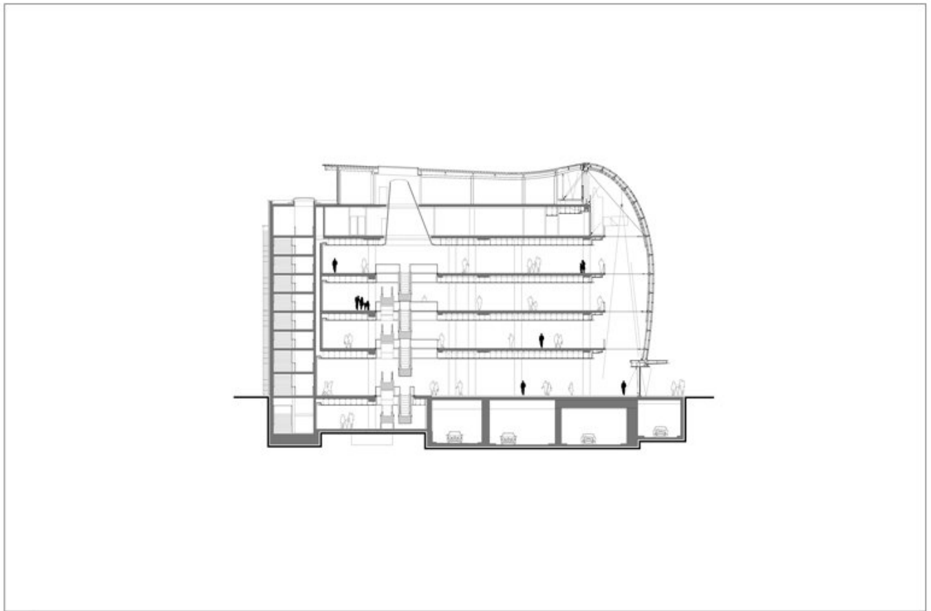
GEBÄUDESCHNITT KAUFHAUS, P & C, KÖLN
