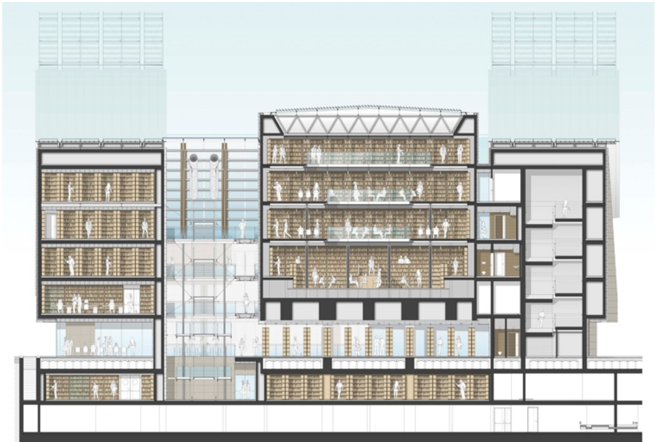
NUOVA BIBLIOTECA UNIVERSITARIA Renzo Piano Building Workshop
